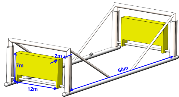
Fig. 15. Sketch of the UM FOSWEC.
